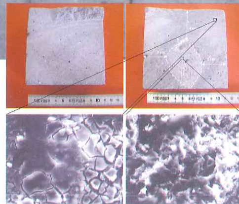
含浸深さ測定試験 [C.S.G.Palladio srl]
